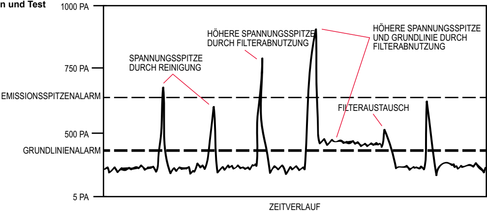
Abbildung 3: Typische Filteremissionen
