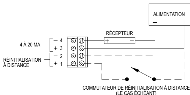
Figure 1 : câblage général pour l'installation (non IS)
