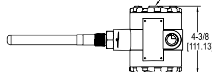
Bague de raccordement mâle NPT 3/4 po (19 mm) ou mâle BSPT 3/4 po (19 mm) 2X ENTRÉE ÉLECTRIQUE 1/2 po (12,7 mm) NPT OU M20
